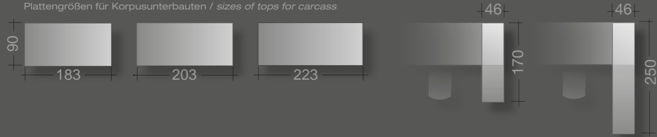
Plattengrößen für Korpusunterbauten / sizes of tops for carcass
